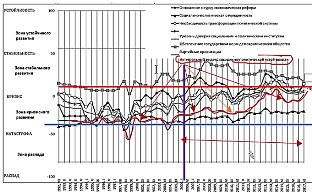
Рисунок 3 - Динамика развития индекса социально-политической устойчивости (1992-2017, красная тенденция)
